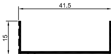
BX-060 0,181 Kg/m
