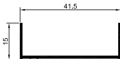
BX-105 0,181 Kg/m
