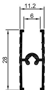
BX-063 0,211Kg/m
