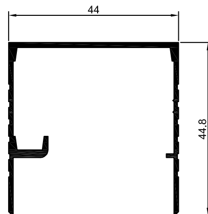
BX-064 0,494 Kg/m
