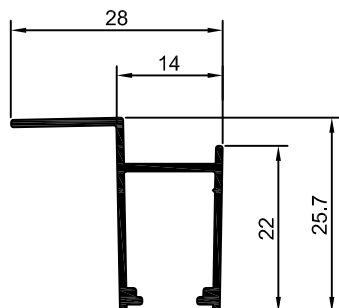
BX-199 0,206 Kg/m
