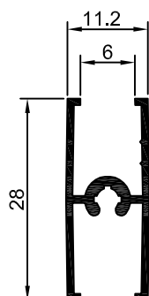
BX-108 0,203 Kg/m
