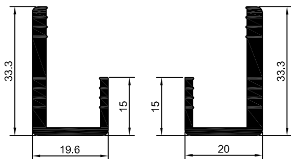
GR-021 0,480 Kg/m
