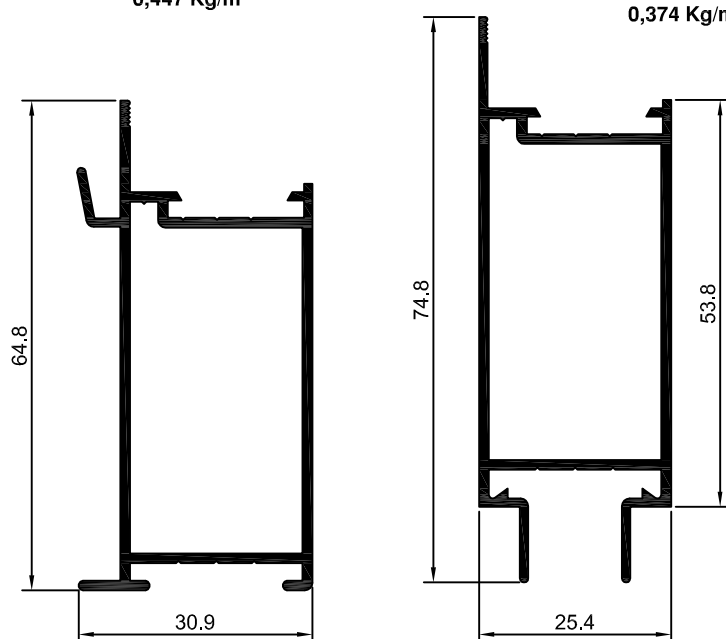
90-243 SU-243 0,664 kg/m
