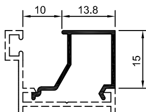
90-103 SU-103 0,138 Kg/m
