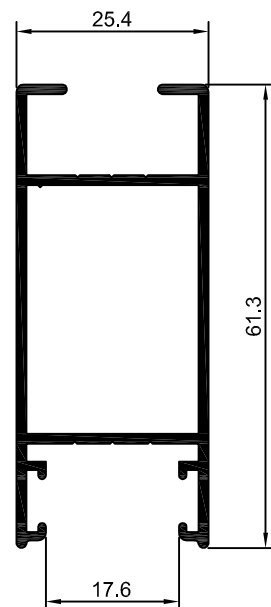
90-238 SU-238 0,669 Kg/m
