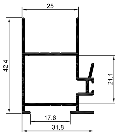
90-556 0,485 Kg/m
