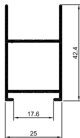
90-072 SU-072 0,401 Kg/m
