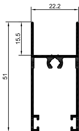
90-187 SU-187 0,466 Kg/m
