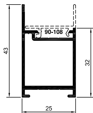
90-120 SU-120 0,447 Kg/m
