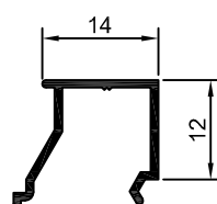
90-202 0,114 kg/m
