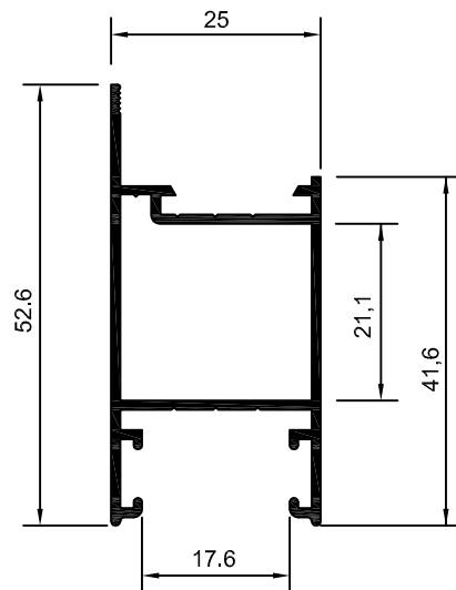
90-039 SU-039 0,472 Kg/m
