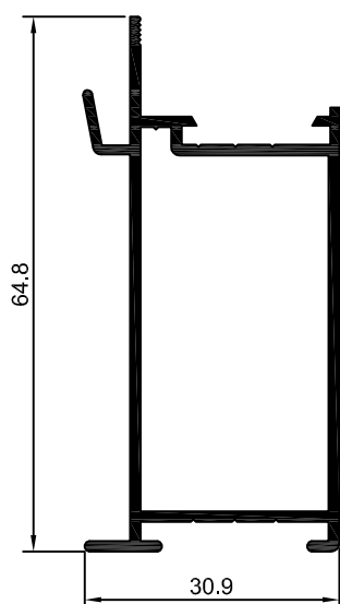
90-243 SU-243 0,664 kg/m
