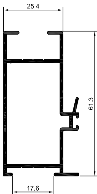
90-239 SU-239 0,734 Kg/m
