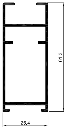
90-241 SU-241 0,697 Kg/m
