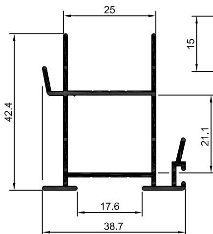
90-069 SU-069 0,524 Kg/m
