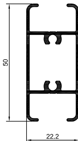
90-188 SU-188 0,580 Kg/m
