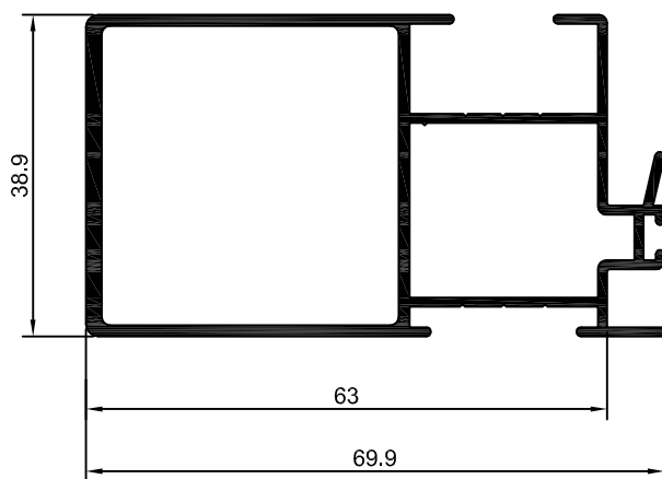
90-061 SU-061 0,981 Kg/m
