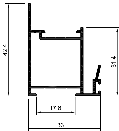
90-041 SU-041 0,462 Kg/m
