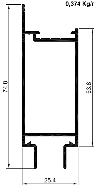
90-244 SU-244 0,683 kg/m
