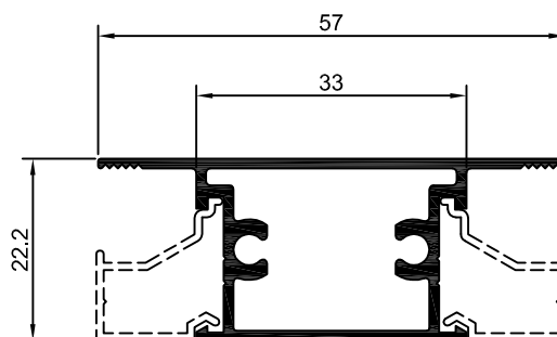
90-227 SU-227 0,540 Kg/m
