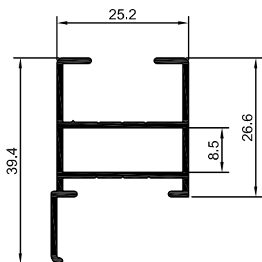
90-090 SU-090 0,382 Kg/m
