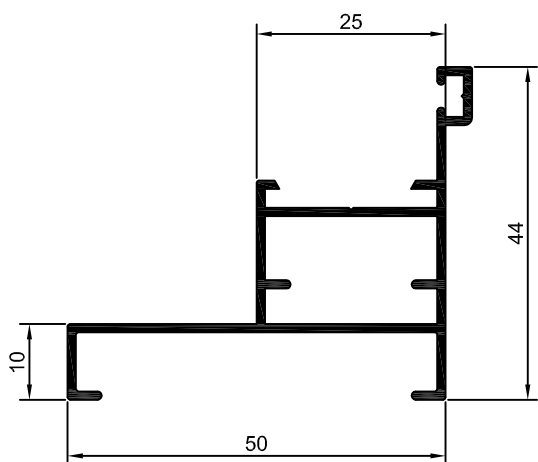
90-089 0,507 Kg/m
