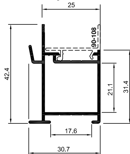
90-040 SU-040 0,435 Kg/m
