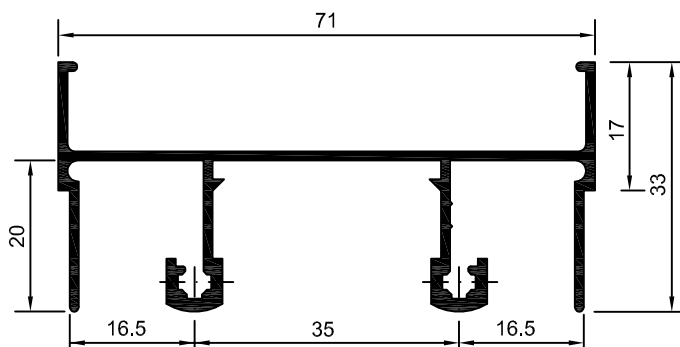
90-001 SU-001 0,715 Kg/m
