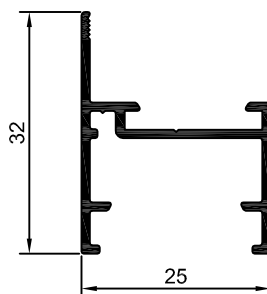
90-088 SU-088 0,271 Kg/m
