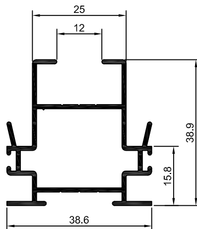
90-057 SU-057 0,583 Kg/m
