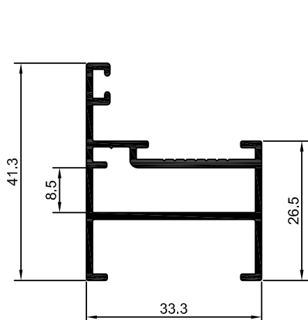
90-279 SU-279 0,534 Kg/m
