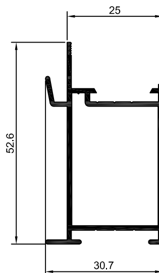
90-282 0,528 Kg/m
