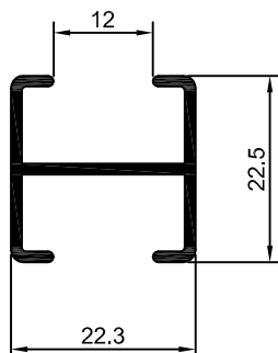
90-285 0,276 Kg/m
