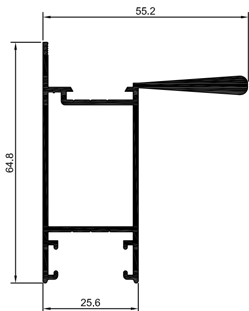
90-280 SU-280 0,911 Kg/m
