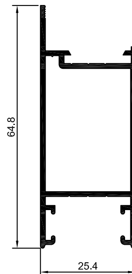
90-245 SU-245 0,634 kg/m
