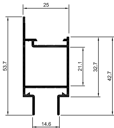
90-192 SU-192 0,475 Kg/m
