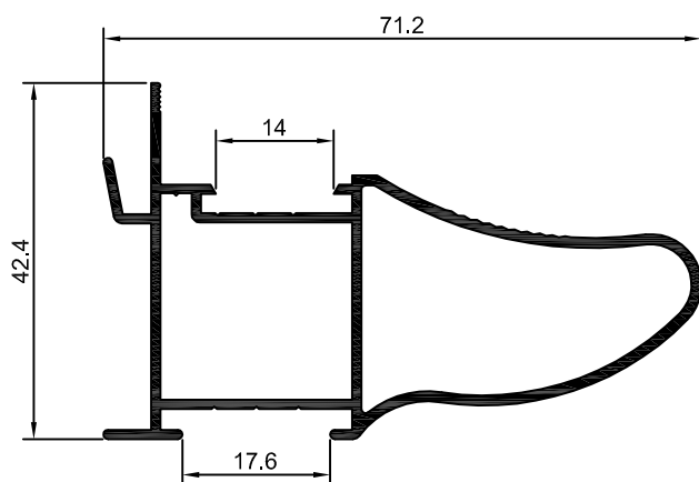
90-140 0,734 Kg/m
