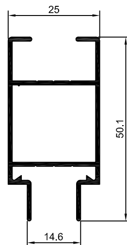
90-190 SU-190 0,499 Kg/m
