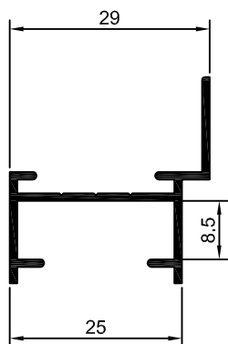
90-071 SU-071 0,255 Kg/m
