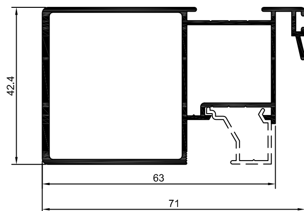
90-049 SU-049 0,969 Kg/m
