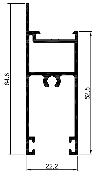
90-246 SU-246 0,642 kg/m
