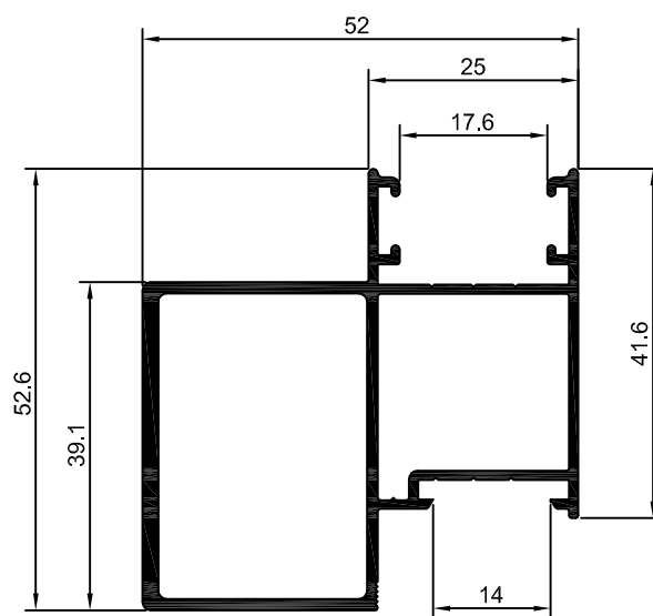
90-044 0,878 Kg/m
