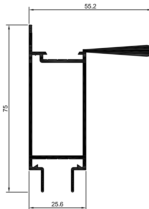
90-281 SU-281 0,976 Kg/m
