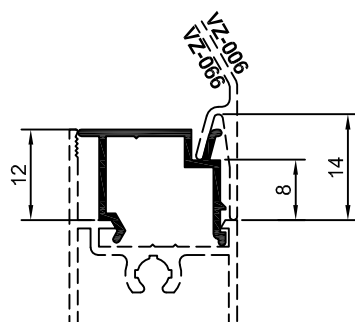
90-203 SU-203 0,133 Kg/m
