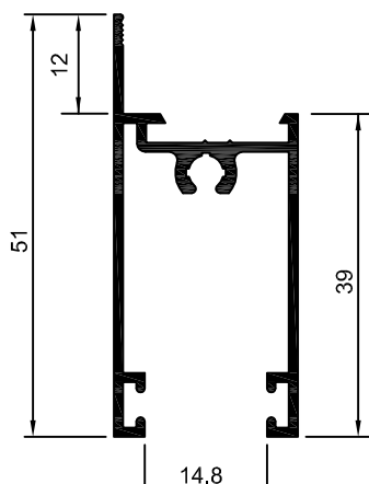
90-053 SU-053 0,437 Kg/m
