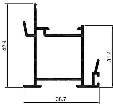
90-042 90-042 0,512 Kg/m
