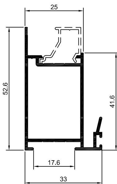
90-283 0,556 Kg/m
