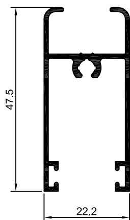
90-186 SU-186 0,455 Kg/m
