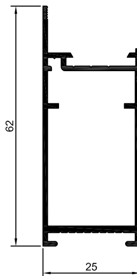
90-111 SU-111 0,599 kg/m
