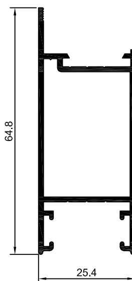
90-245 SU-245 0,634 kg/m
