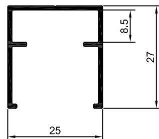
90-093 SU-093 0,260 Kg/m
