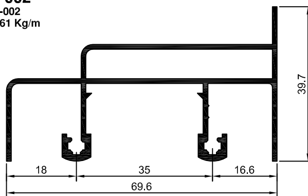
90-205 0,854 Kg/m
