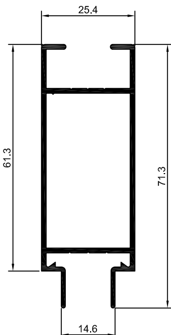
90-240 SU-240 0,724 Kg/m
