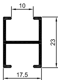
90-286 0,214 Kg/m
