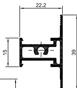
DS-520 0,381 Kg/m
