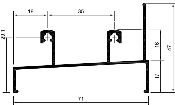
90-002 SU-002 0,661 Kg/m
