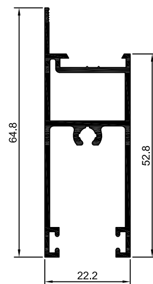
90-246 SU-246 0,642 kg/m
