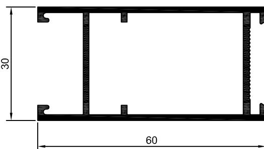
30-077 30-077 0,791 kg/m
