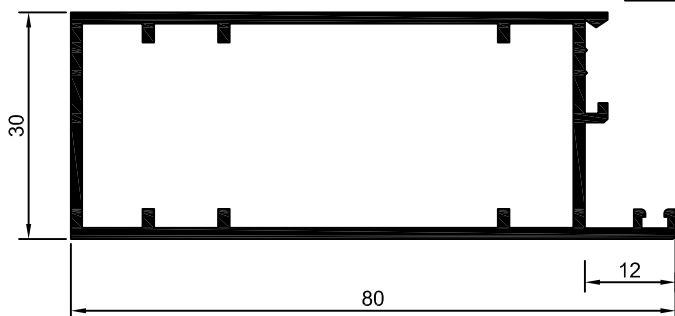
30-033 30-033 0,924 Kg/m
