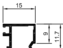
30-110 BG-010 0,109 Kg/m
