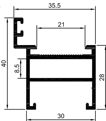
30-023 30-023 0,561 Kg/m
