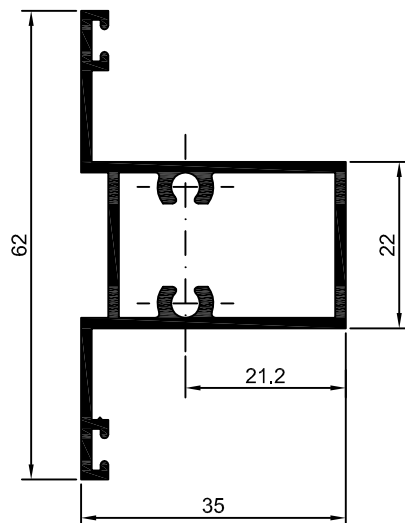
30-235 30-235 0,694 Kg/m
