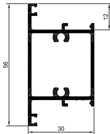
30-025 30-025 0,721 Kg/m
