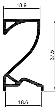
MV-061 0,374 Kg/m
