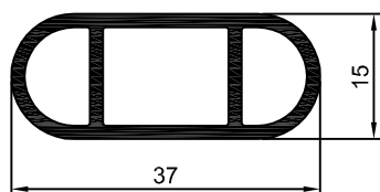
MV-013 0,477 Kg/m
