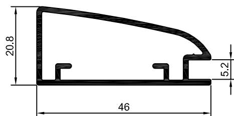
MV-114 0,488 Kg/m
