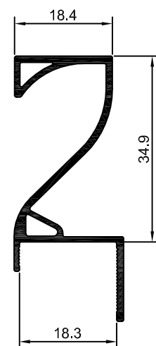
MV-088 0,382 Kg/m
