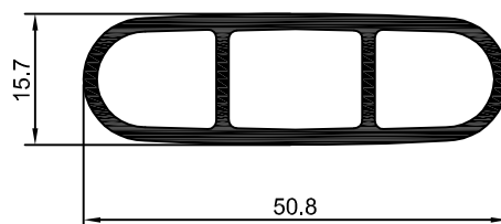
DS-834 0,626 Kg/m
