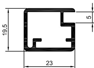
MV-010 0,363 Kg/m
