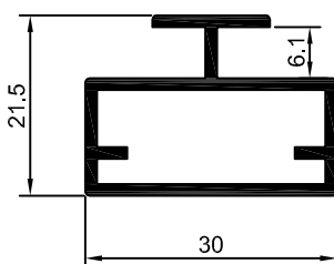
MV-019 0,415 Kg/m
