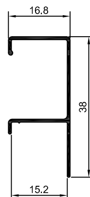
MV-095 0,168 Kg/m
