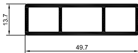
MV-059 0,528 Kg/m
