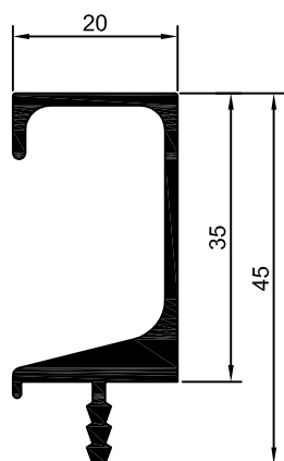
MV-012 0,512 Kg/m
