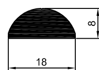
MV-035 0,304 Kg/m
