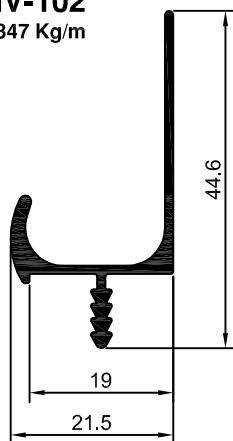
MV-087 0,290 Kg/m
