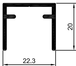
MV-049 0,266 Kg/m
