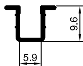
MV-073 0,079 Kg/m
