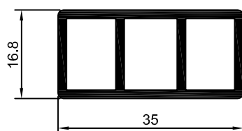
DS-839 0,537 Kg/m
