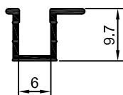
MV-033 0,089 Kg/m
