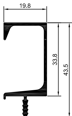
MV-089 0,379 Kg/m
