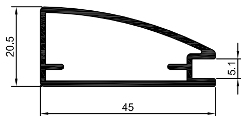
MV-001 0,499 Kg/m
