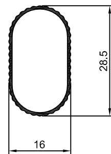
MV-070 0,141 Kg/m
