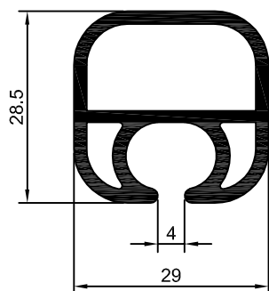
DS-915 0,721 Kg/m
