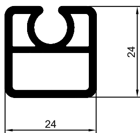
MV-032 0,572 Kg/m
