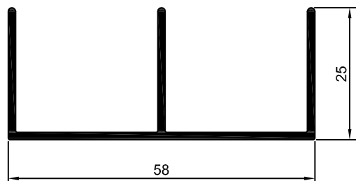
MV-036 0,488 Kg/m
