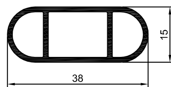
MV-056 0,401 Kg/m
