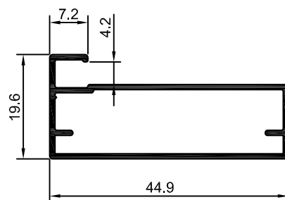
MV-082 0,360 Kg/m
