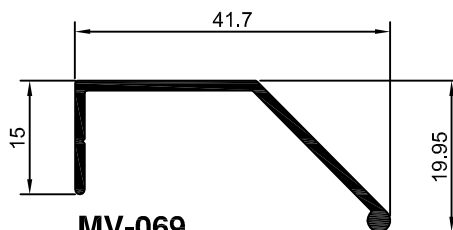
MV-069 0,233 Kg/m
