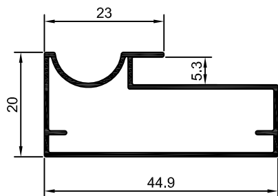
MV-093 0,317 Kg/m
