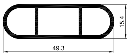
MV-053 0,534 Kg/m
