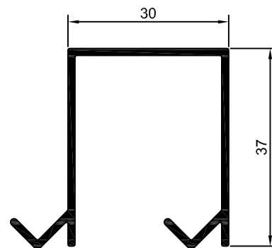
MV-034 0,461 Kg/m
