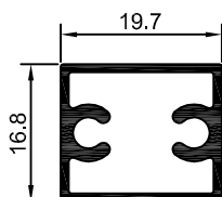
MV-110 0,287 Kg/m
