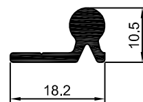
MV-050 0,192 Kg/m
