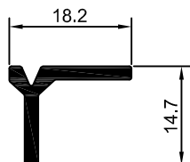
MV-081 0,171 Kg/m
