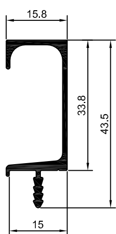
MV-099 0,322 Kg/m
