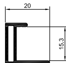
MV-067 0,231 Kg/m
