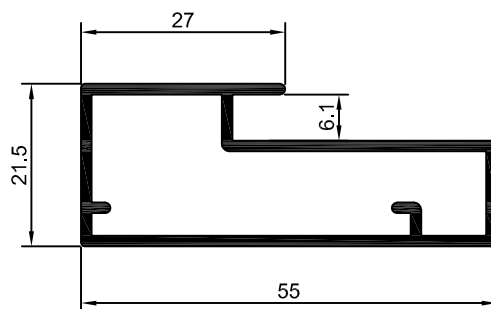
MV-020 0,618 kg/m
