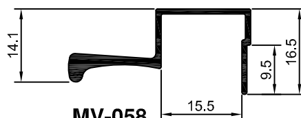
MV-058 0,230 Kg/m
