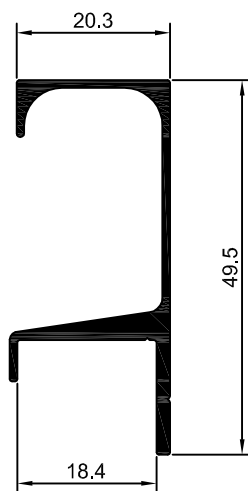
MV-092 0,415 Kg/m
