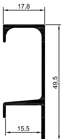
MV-102 0,347 Kg/m
