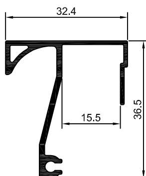
MV-060 0,382 Kg/m
