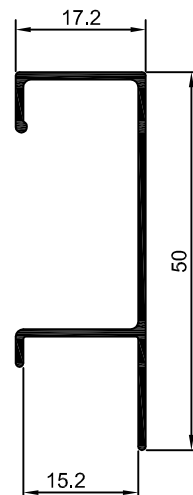
MV-065 0,255 Kg/m
