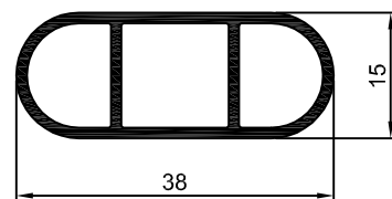
MV-076 0,388 Kg/m
