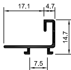
25-118 ME-043 0,130 Kg/m
