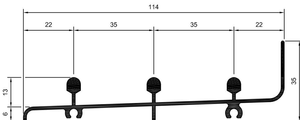
25-112 ME-052 0,956 Kg/m
