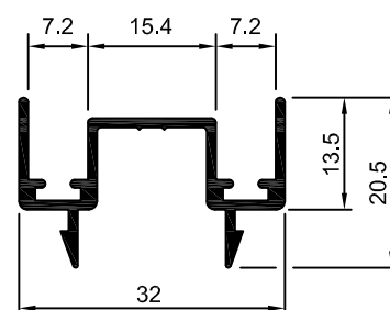
25-114 ME-050 0,305 Kg/m
