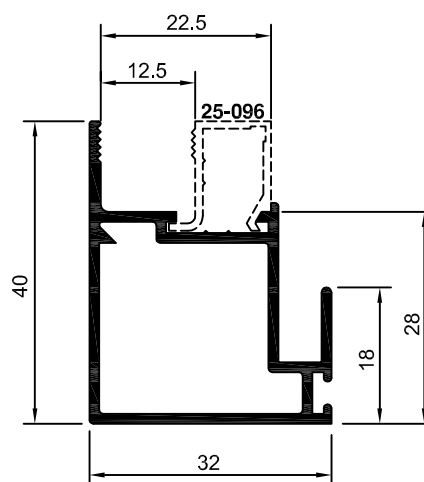
25-120 ME-003 0,448 Kg/m
