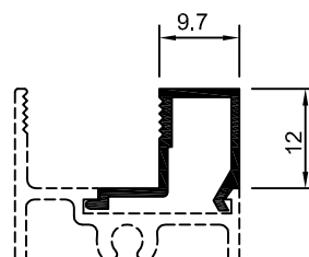
30-012 ME-086 0.132 Kg/m
