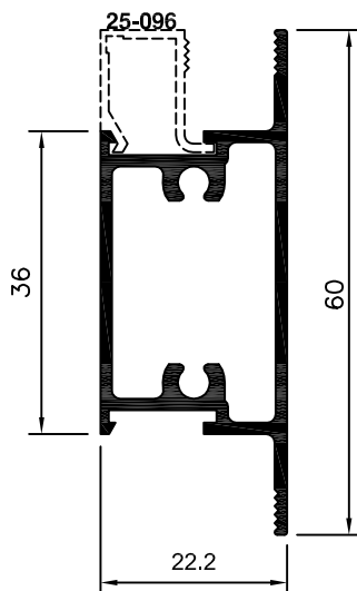
25-100 ME-027 0,620 Kg/m
