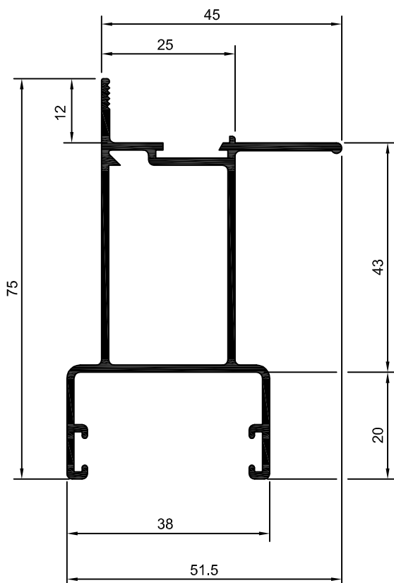
25-035 ME-026 0,872 Kg/m
