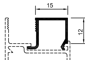
30-011 ME-079 0,132 Kg/m
