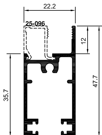
25-102 ME-001 0,537 Kg/m
