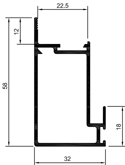
25-034 ME-006 0,653 Kg/m
