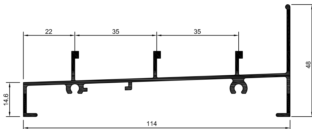
25-138 ME-017 0,983 Kg/m
