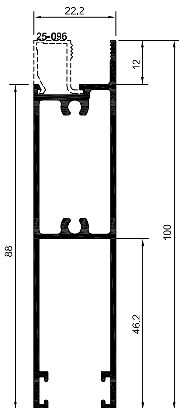
25-101 ME-009 0,988 Kg/m
