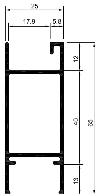
25-098 ME-030 0,697 Kg/m
