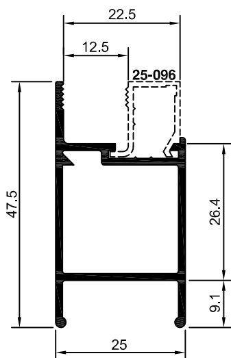
25-119 ME-040 0,429 Kg/m
