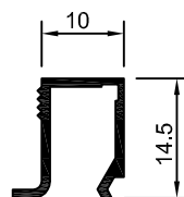
25-096 ME-028 0,103 Kg/m
