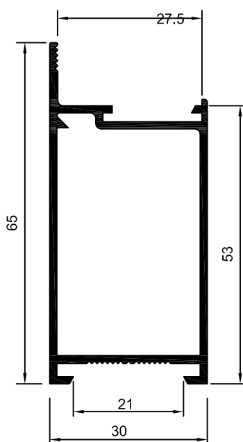
30-015 ME-075 0,672 Kg/m
