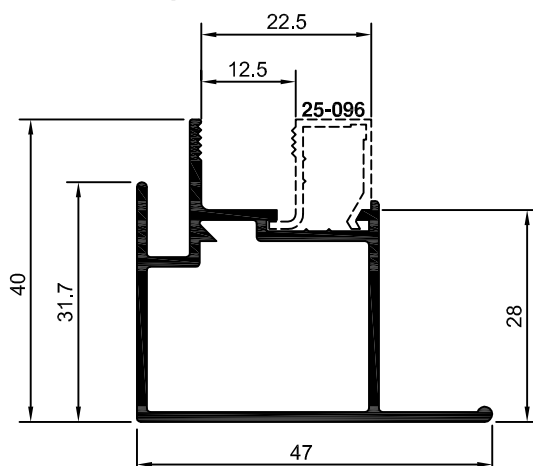
25-122 ME-004 0,472 Kg/m
