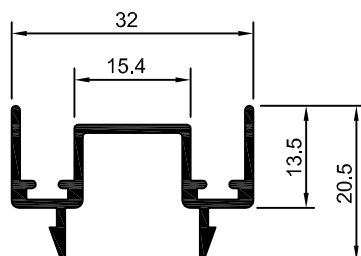
25-114 ME-050 0,305 Kg/m
