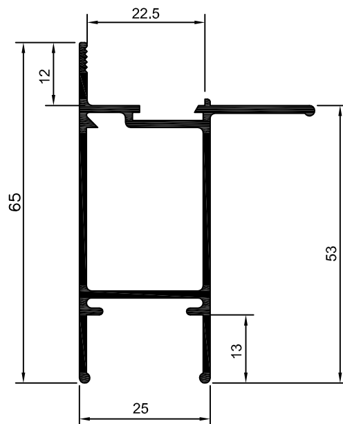
25-037 ME-008 0,734 Kg/m
