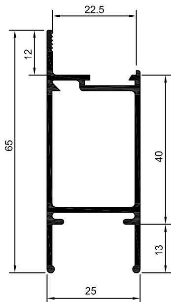
25-033 ME-025 0,653 Kg/m
