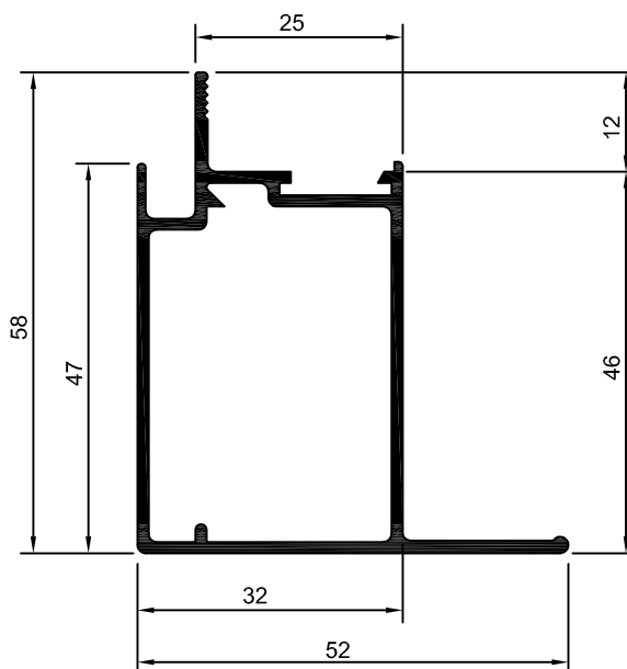
25-036 ME-007 0,735 Kg/m
