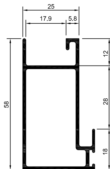
25-099 ME-031 0,699 Kg/m
