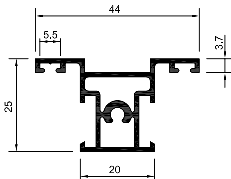
25-048 MM-376 0,521 Kg/m
