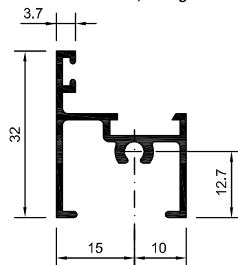
25-046 25-312 0,350 Kg/m
