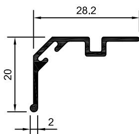
25-047 ME-056 0,184 Kg/m
