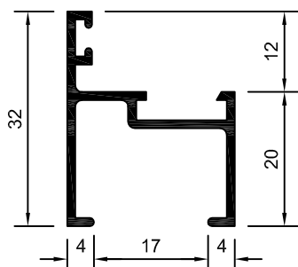
25-045 25-311 0,305 Kg/m
