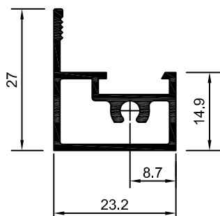
25-049 25-301 0,343 Kg/m
