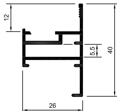
25-052 MM-375 0,389 Kg/m
