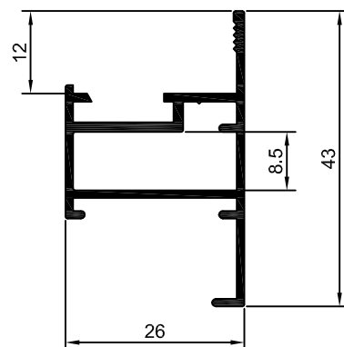
25-315 25-315 0,407 Kg/m
