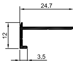
25-377 MM-377 0,119 Kg/m
