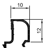
20-102 0,106 Kg/m
