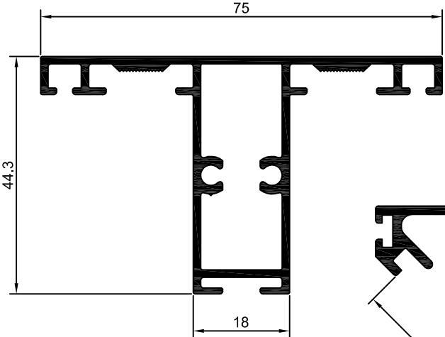
FC-231 FC-231 0,986 Kg/m
