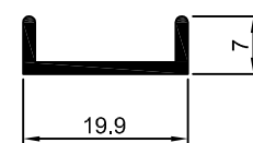
PU-061 0,120 kg/m
