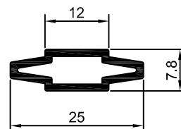
DS-129 0,200 Kg/m
