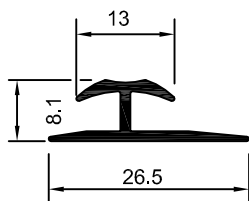
DS-170 DS-285 0,143 Kg/m
