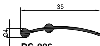
DS-336 0,149 kg/m
