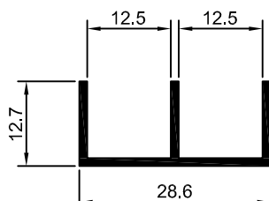
DS-772 0,206 Kg/m
