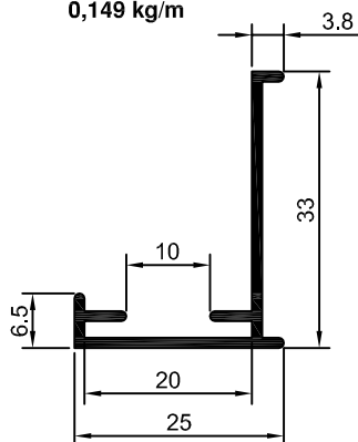
DS-183 0,240 kg/m
