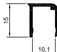
DS-882 0,133 Kg/m
