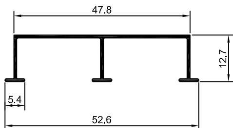
DS-775 0,211 Kg/m
