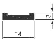
DS-418 0,086 Kg/m
