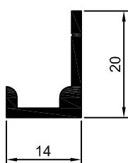
DS-824 0,198 Kg/m
