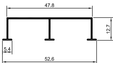
DS-775 0,211 Kg/m
