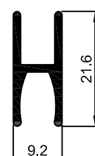
DS-119 0,192 Kg/m
