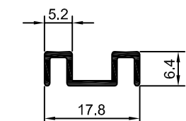
DS-709 DS-1099 DS-294 DS-294 0,130 kg/m 0,106 kg/m
