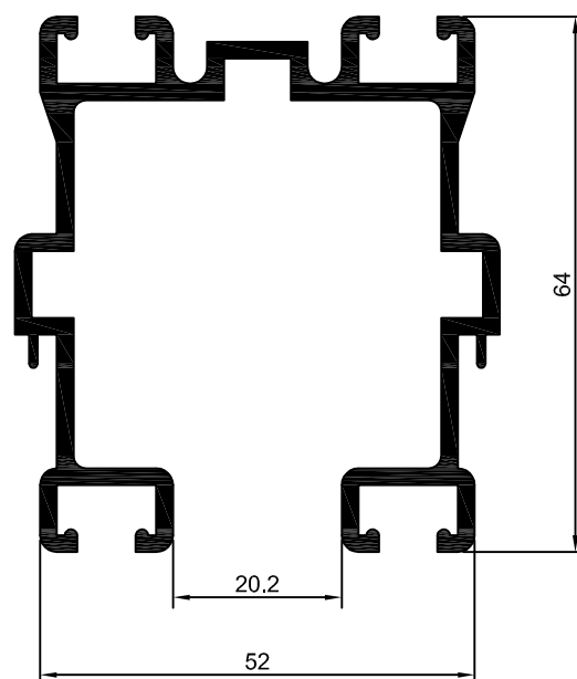
DS-330 1,585 Kg/m
