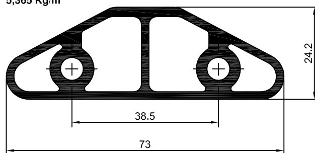
DS-563 1,523 Kg/m
