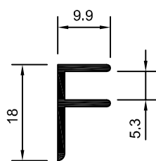
DS-168 0,121 Kg/m
