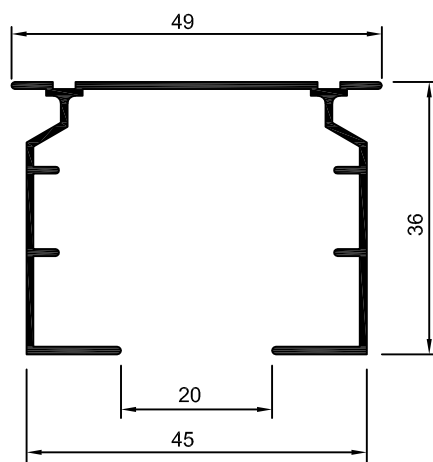
DS-271 0,402 Kg/m
