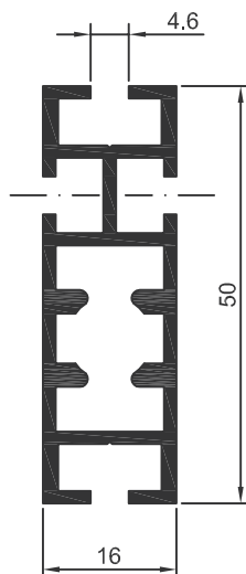
DS-568 0,754 Kg/m
