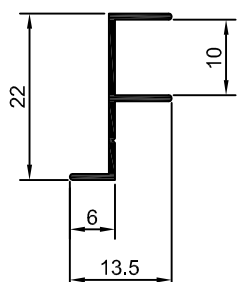
DS-535 0,089 Kg/m
