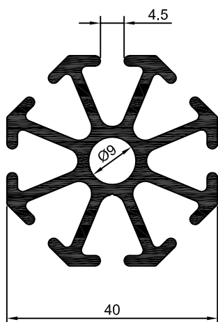
DS-569 1,253 Kg/m
