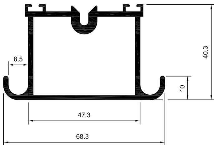
DS-163 1,318 Kg/m
