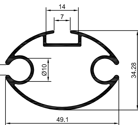
DS-1021 0,626 Kg/m PÁG.68-05
