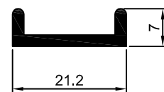
PU-051 0,173 kg/m
