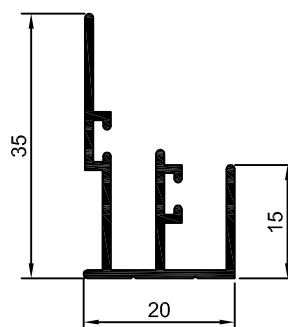
DS-080 0,290 Kg/m
