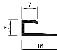
DS-385 0,071 Kg/m
