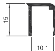
DS-882 0,133 Kg/m
