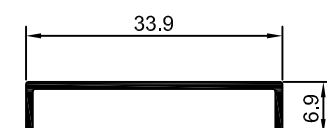
PU-069 0,111 Kg/m
