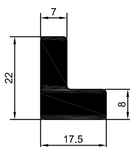
CT-050 0,642 kg/m
