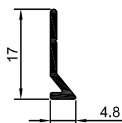
DS-743 0,070 kg/m
