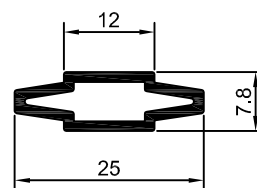
DS-129 0,200 Kg/m
