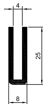
PU-053 0,287 Kg/m
