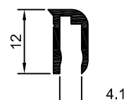
DS-884 0,092 Kg/m
