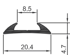
DS-770 0,100 Kg/m
