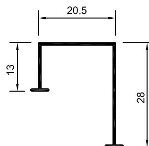
DS-169 0,130 Kg/m
