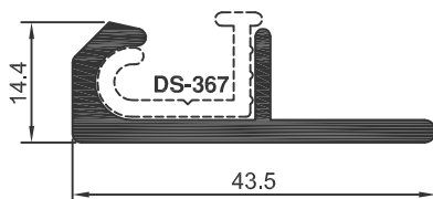
DS-368 0,489 Kg/m
