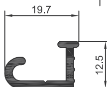
DS-367 0,208 Kg/m
