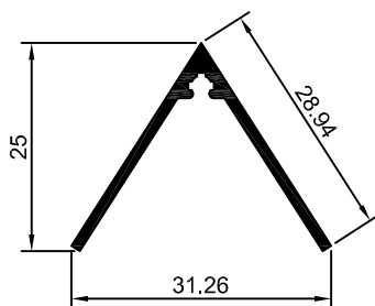
DS-237 0,197 kg/m
