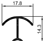
DS-1504 0,092 Kg/m
