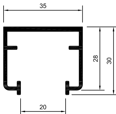
DS-075 0,513 Kg/m
