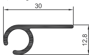
DS-590 0,217 Kg/m
