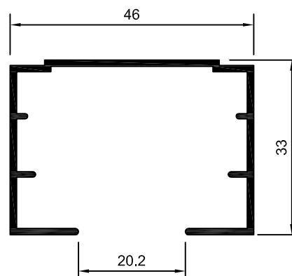
DS-014 BK-772 0,459 Kg/m
