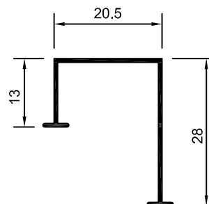
DS-169 0,130 Kg/m
