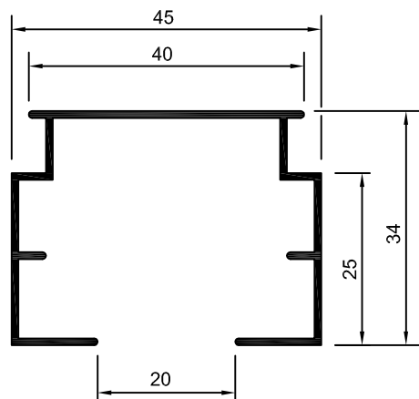
DS-155 0,394 Kg/m
