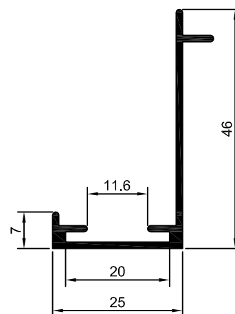
DS-181 0,313 kg/m
