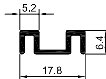
DS-709 DS-294 0,130 kg/m
