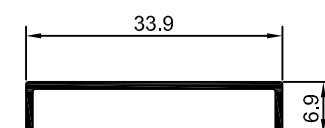
PU-069 0,111 Kg/m
