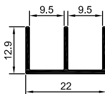
DS-1539 0,157 Kg/m
