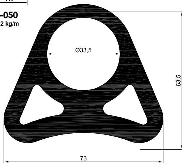
DS-260 5,365 Kg/m
