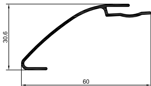
DS-0089 0,319 kg/m
