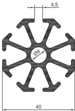
DS-569 1,253 Kg/m
