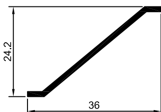
DS-145 0,162 kg/m
