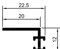
DS-773 0,138 Kg/m
