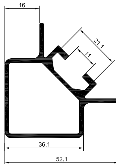
DS-589 0,954 Kg/m
