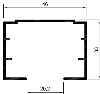
DS-014 BK-772 0,459 Kg/m
