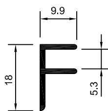
DS-168 0,121 Kg/m
