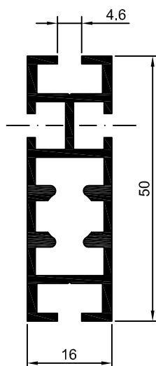
DS-568 0,754 Kg/m
