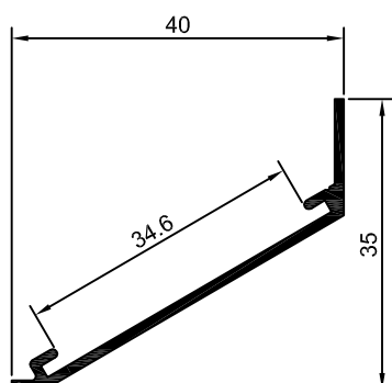
DS-744 0,206 kg/m
