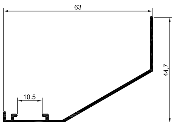
DS-745 0,306 kg/m
