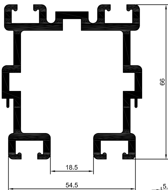
DS-065 2,360 Kg/m
