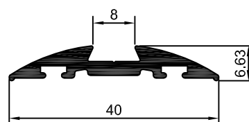
DS-885 0,325 Kg/m
