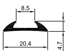
DS-770 0,100 Kg/m
