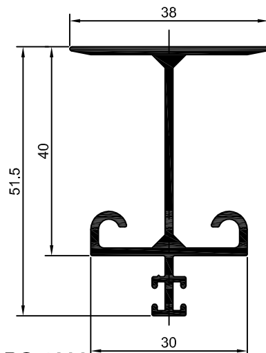
DS-1396 GE-636 0,634 Kg/m
