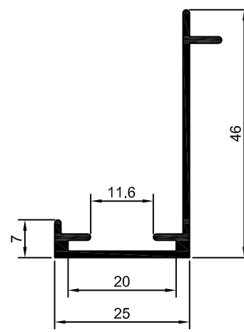
DS-181 0,313 kg/m
