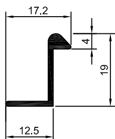
DS-611 0,141 Kg/m
