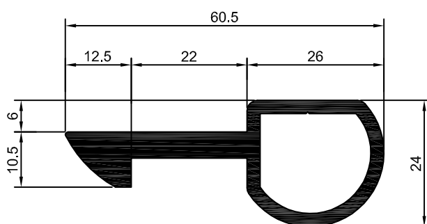
DS-654 1,079 Kg/m
