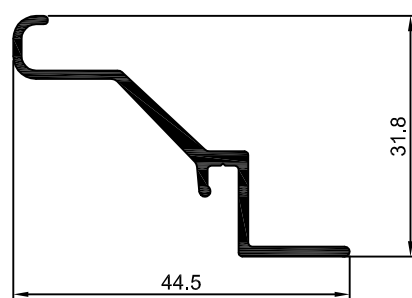
DS-497 0,273 Kg/m
