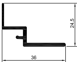
DS-495 0,270 Kg/m
