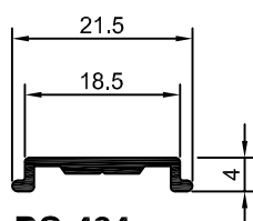
DS-484 0,100 Kg/m
