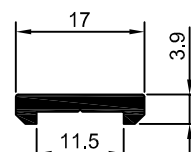
DS-653 0,125 Kg/m
