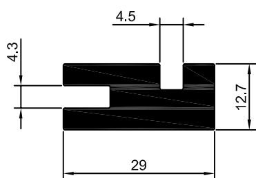
DS-540 0,829 Kg/m
