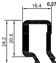
DS-529 0,437 Kg/m
