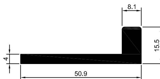
DS-1157 0,802 Kg/m
