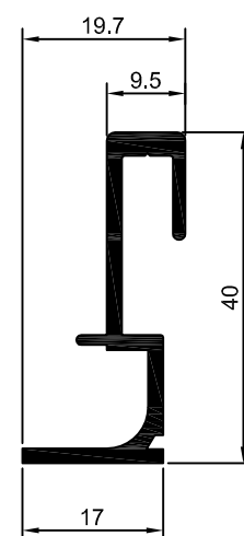
DS-715 0,412 Kg/m
