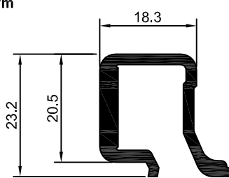
DS-530 0,462 Kg/m
