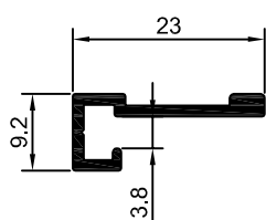
DS-651 0,152 Kg/m
