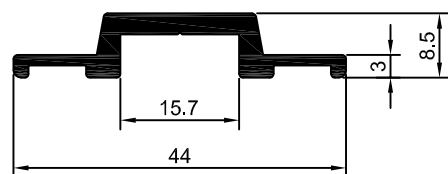
DS-655 0,360 Kg/m
