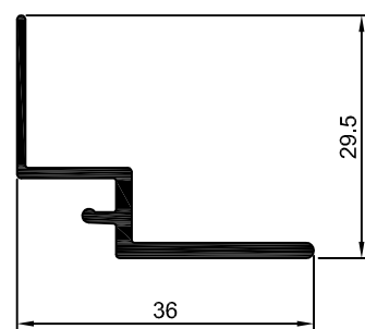
DS-494 0,275 Kg/m
