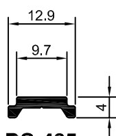
DS-485 0,081 Kg/m
