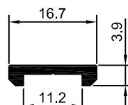
DS-650 0,106 Kg/m
