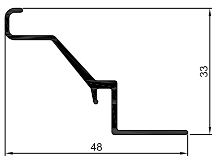
DS-496 0,265 Kg/m
