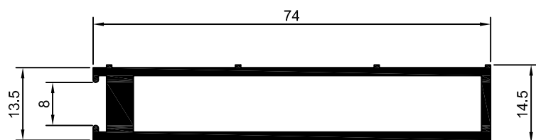
DS-576 0,810 Kg/m
