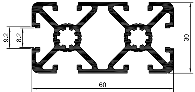
DS-1219 1,504 Kg/m
