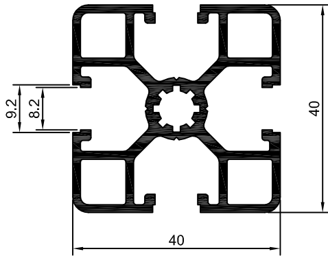
DS-1050 1,171 Kg/m
