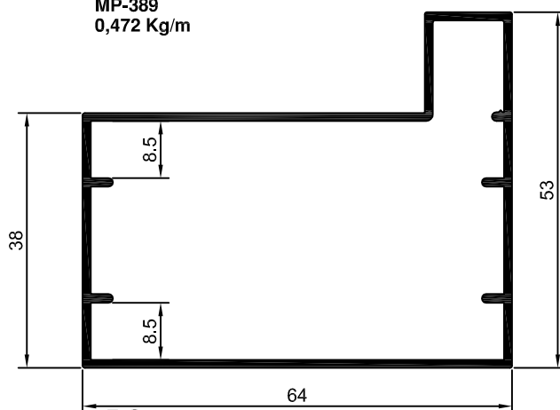
DS-1319 0,797 Kg/m
