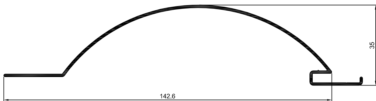
LB-012 0,618 Kg/m
