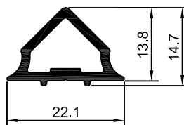
30-044 30-044 0,225 Kg/m
