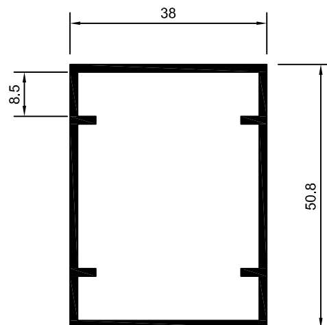
DS-007 DS-827 DS-1097 PC-004 PC-004 PC-004 0,751 Kg/m 0,659 Kg/m 0,561 Kg/m
