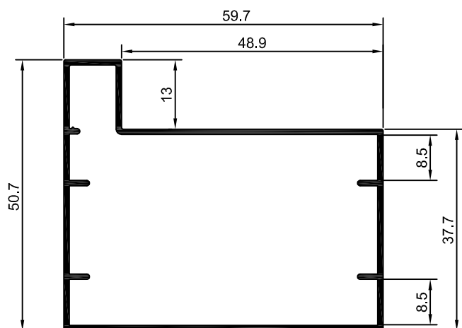
DS-1503 0,631 Kg/m
