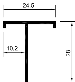
DS-226 CM-008 0,178 Kg/m
