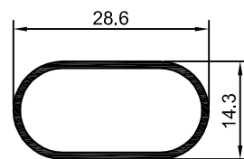
DS-1336 0,157 Kg/m
