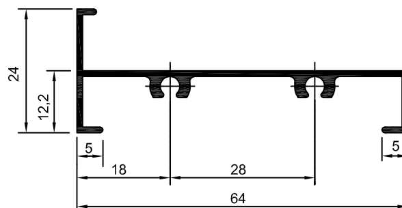
20-080 MP-389 0,472 Kg/m
