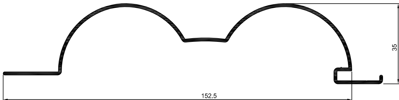
LB-004 0,840 Kg/m
