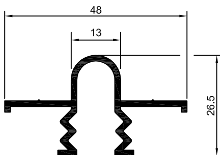
DS-044 DS-844 PC-006 PC-006 0,456 Kg/m 0,366 Kg/m
