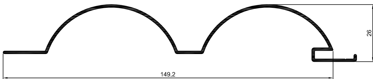
LB-248 0,740 Kg/m
