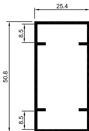
DS-173 0,508 Kg/m
