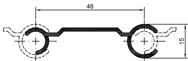
DS-227 0,375 Kg/m
