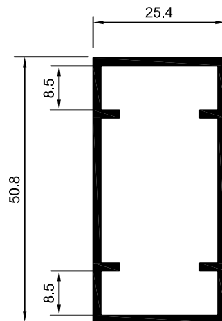
DS-005 PC-002 0,650 Kg/m
