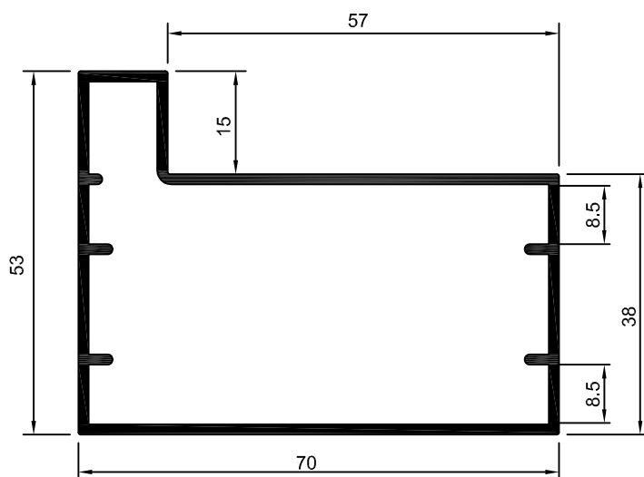
DS-199 PC-010 1.031 Kg/m
