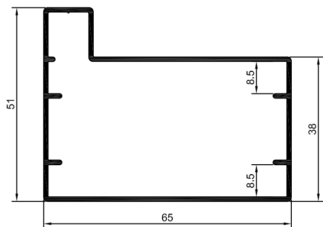
DS-1429 0,770 Kg/m
