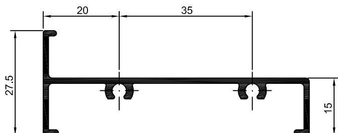
25-517 25-517 0,531 Kg/m
