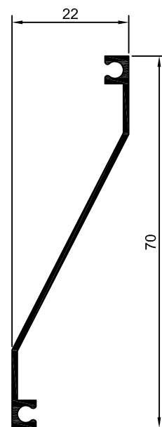
28-515 28-515 0,252 Kg/m
