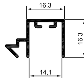
DS-1391 0,217 Kg/m
