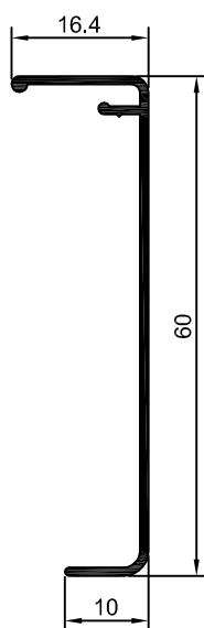
BX-181 0,241 kg/m
