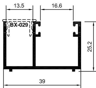
BX-027 2935 0,424 Kg/m
