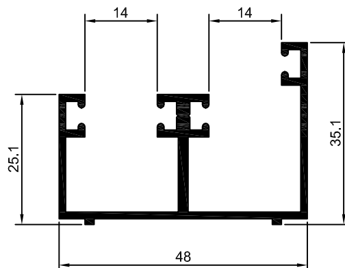
BX-150 0,650 Kg/m
