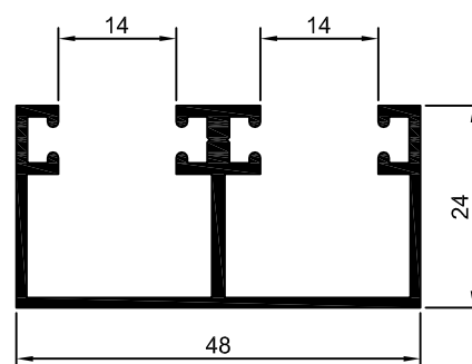
BX-170 0,561 Kg/m
