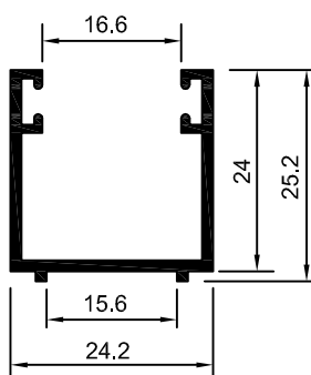
BX-054 2936 0,292 Kg/m
