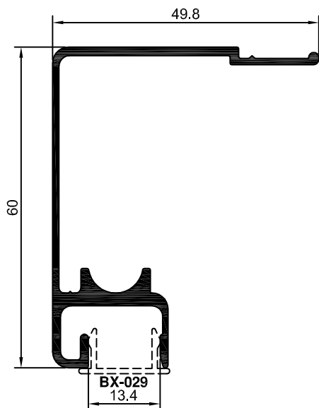
BX-180 0,680 kg/m
