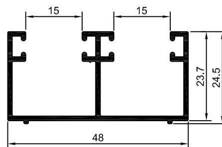
BX-210 0,504 Kg/m
