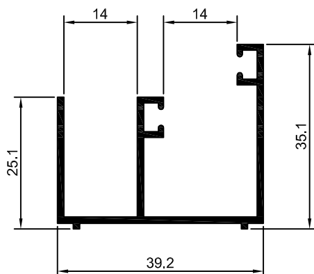
BX-141 0,447 Kg/m
