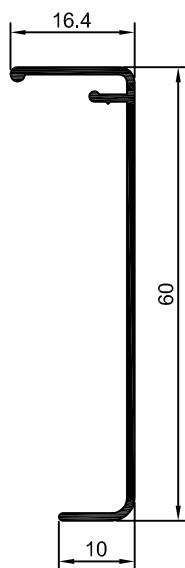
BX-181 0,241 kg/m
