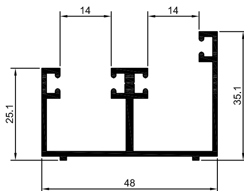
BX-150 0,650 Kg/m
